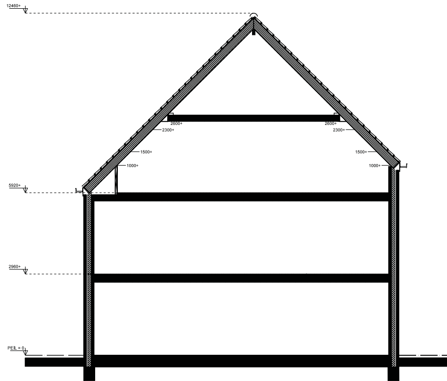
DOORSNEDE type D3
