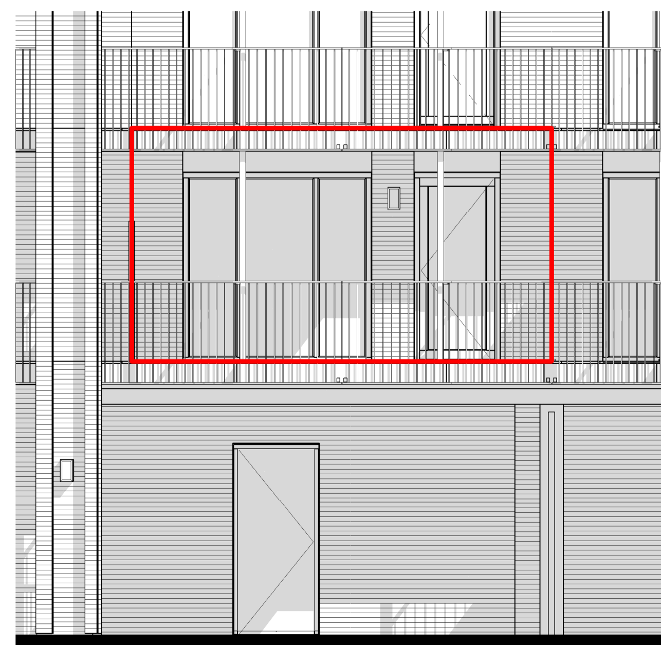
binnengevel (Zuid)
