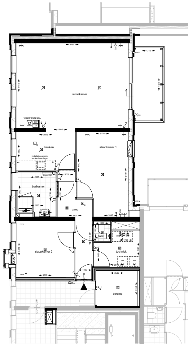
plattegrond 1 : 50
