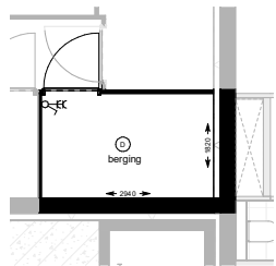
eerste verdieping 1 : 50
