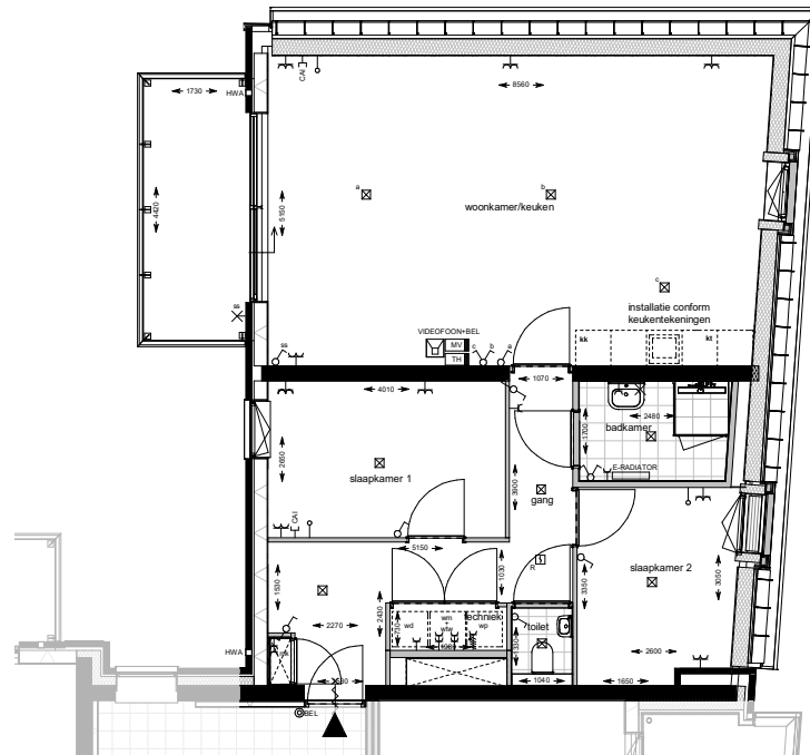
derde verdieping 1 : 50
