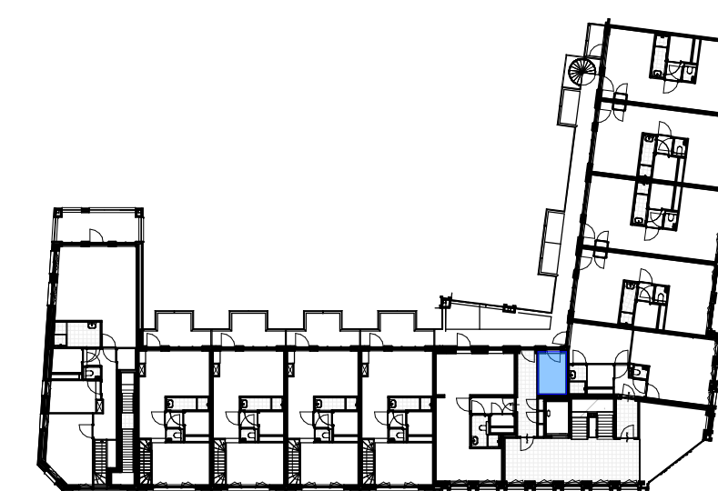
1e verdieping
