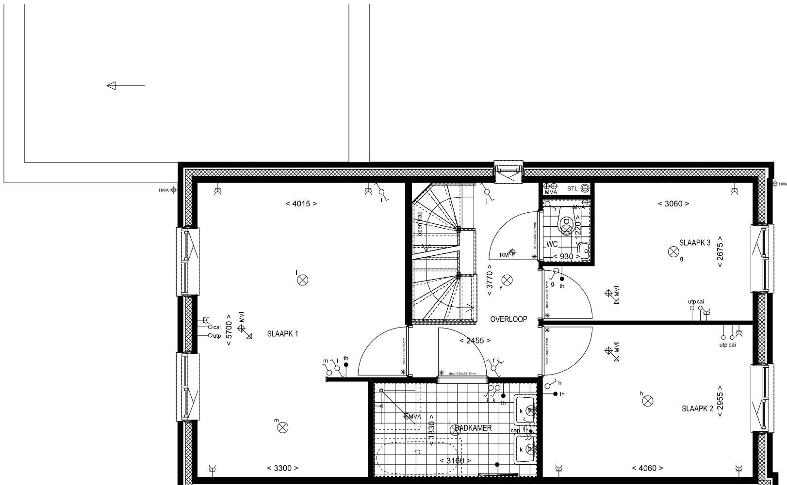
1e VERDIEPING BNR 10 TYPE D1sp
