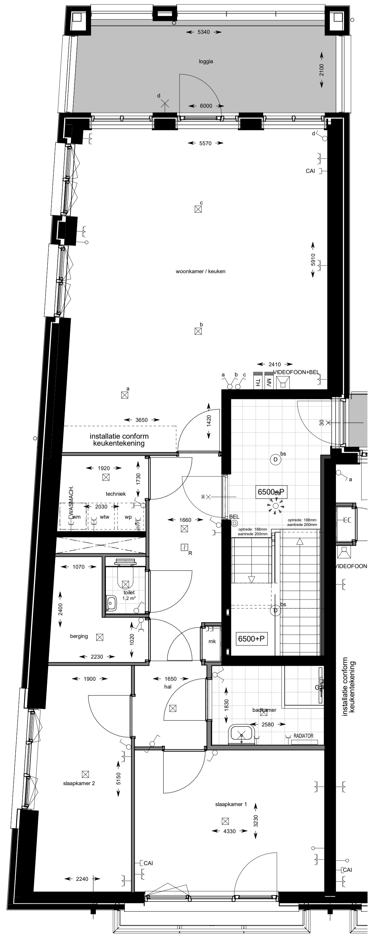
tweede verdieping
