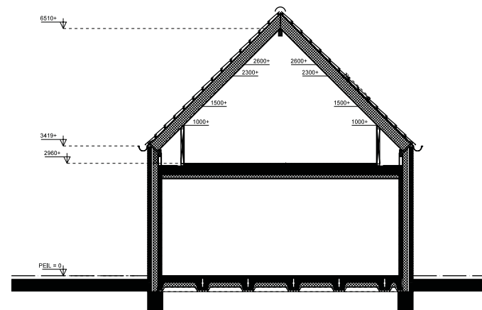
DOORSNEDE
