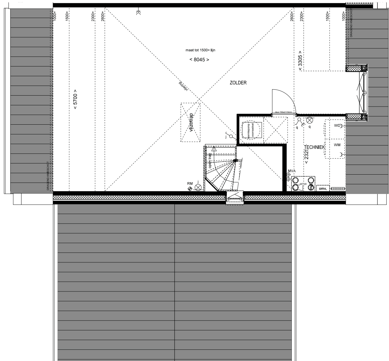
2e VERDIEPING BNR 7 TYPE E2
