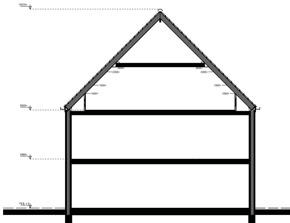
DOORSNEDE type E2
