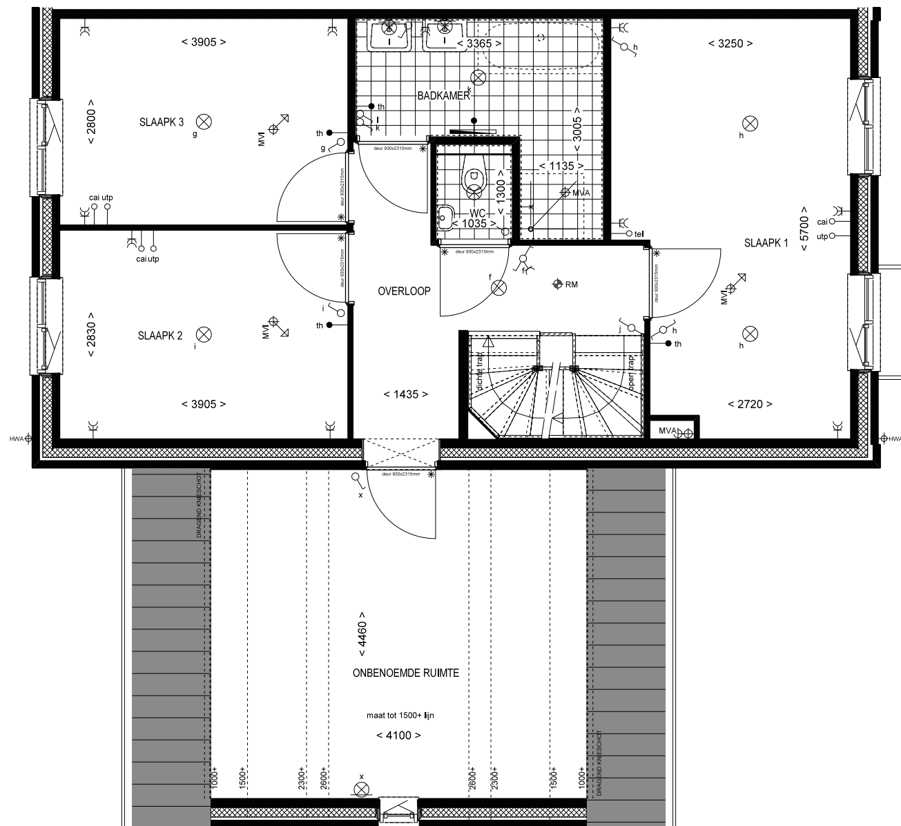
1e VERDIEPING BNR 7 TYPE E2
