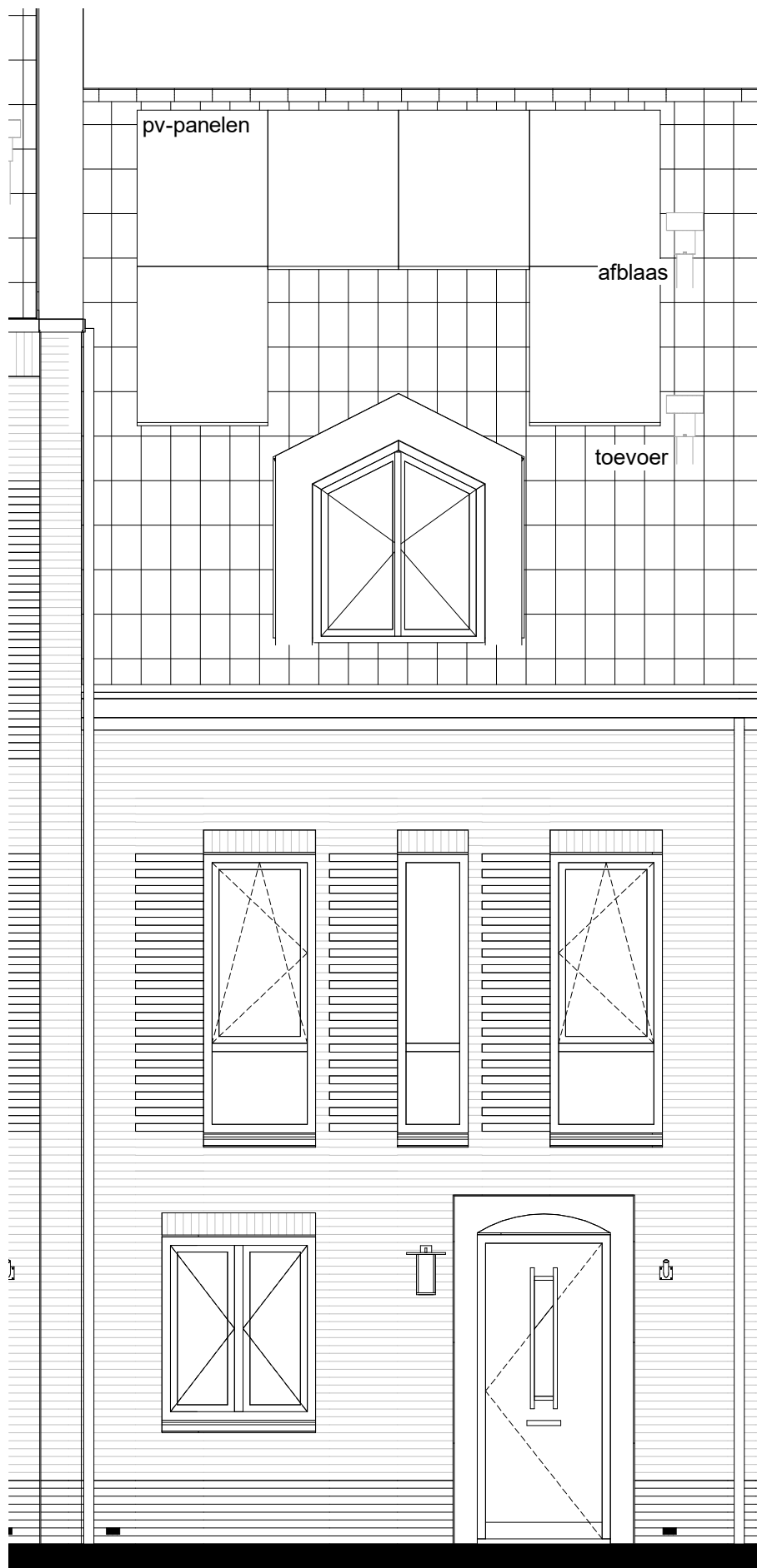
voorgevel
