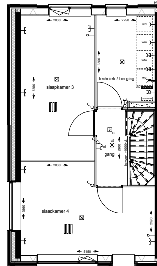
tweede verdieping 1 : 50
