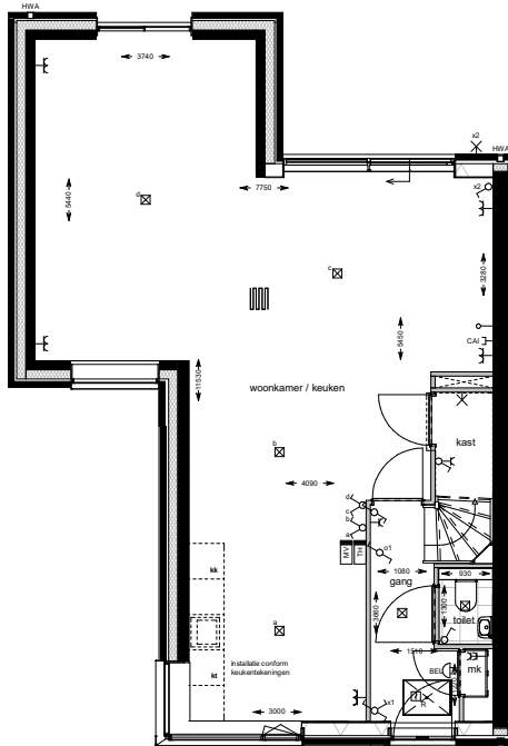
begane grond 1 : 50
