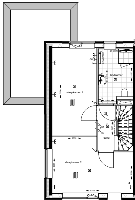
eerste verdieping 1 : 50
