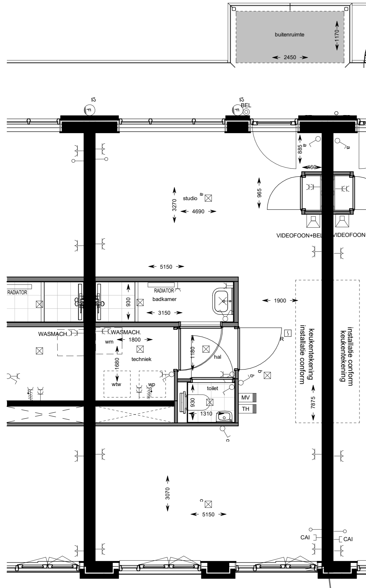
derde verdieping
