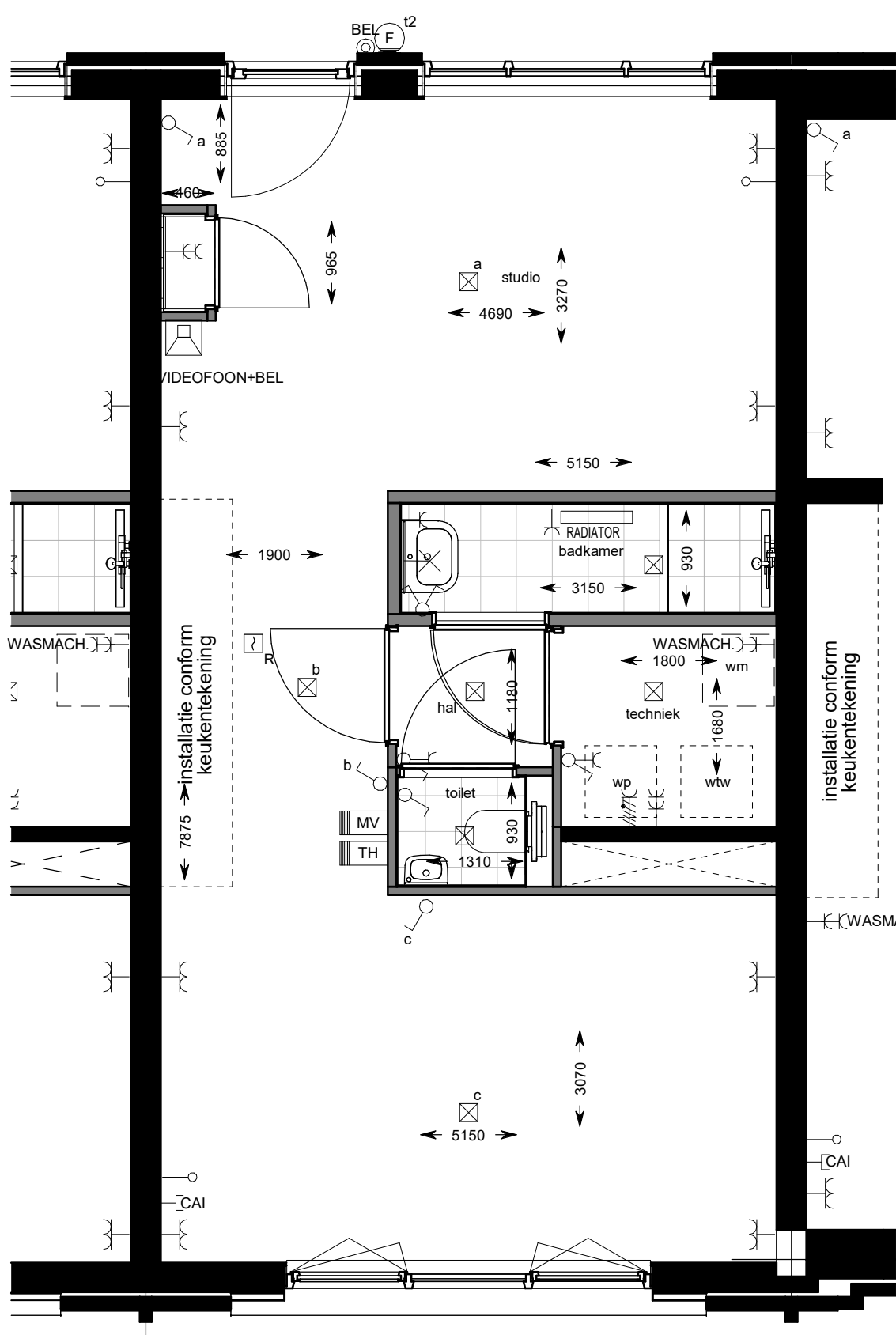
vierde verdieping
