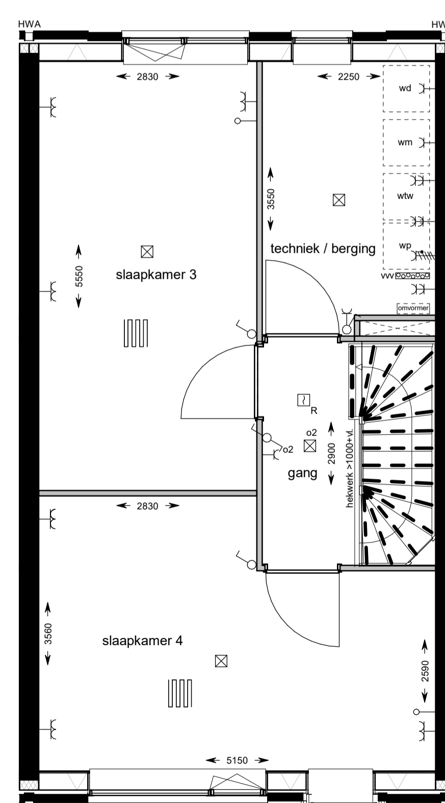
tweede verdieping 1 : 50
