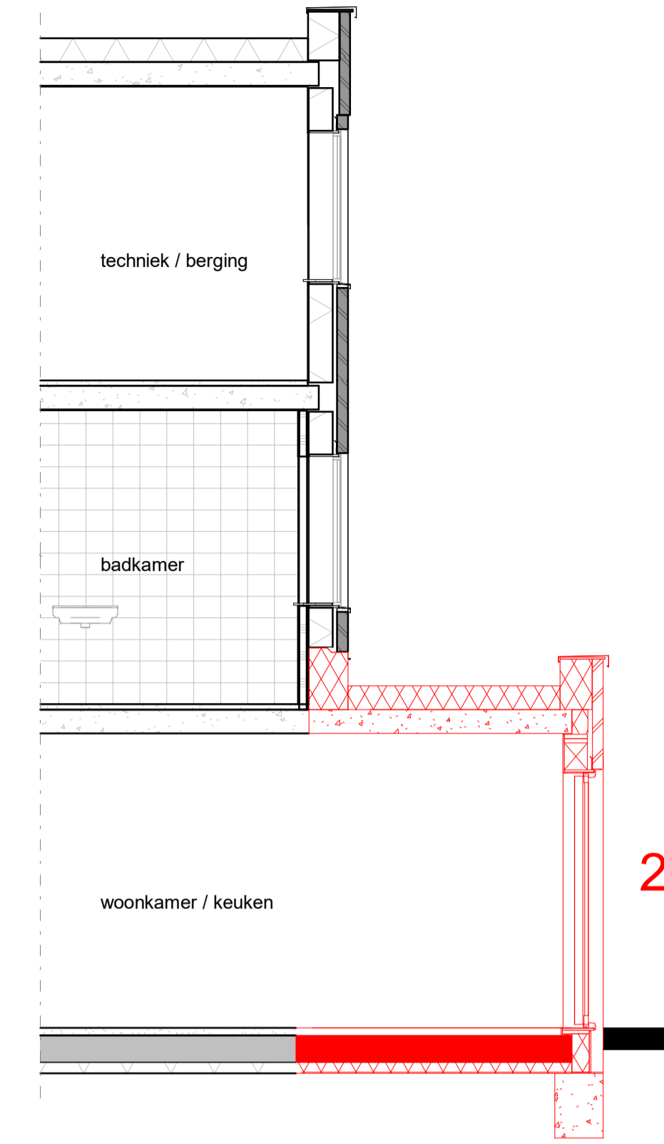
doorsnede B
