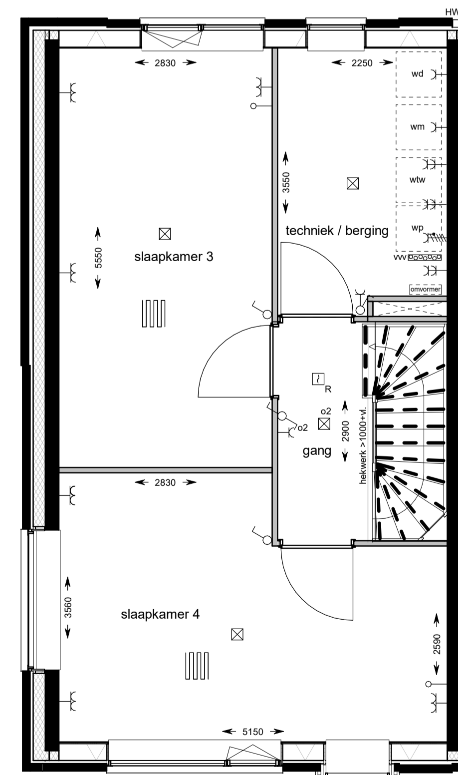
tweede verdieping 1 : 50
