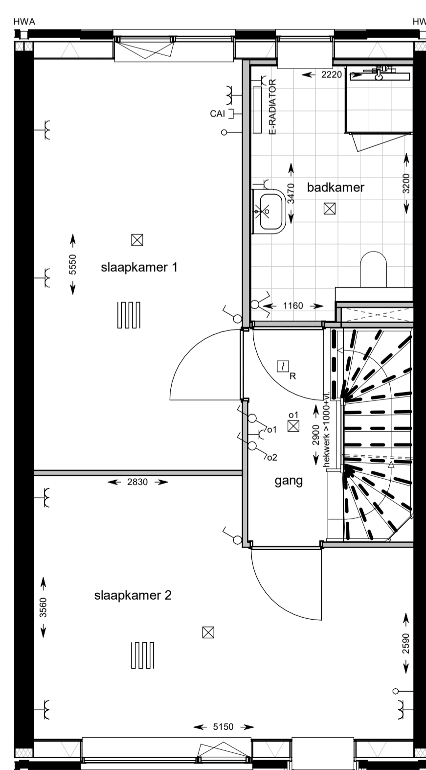
eerste verdieping 1 : 50
