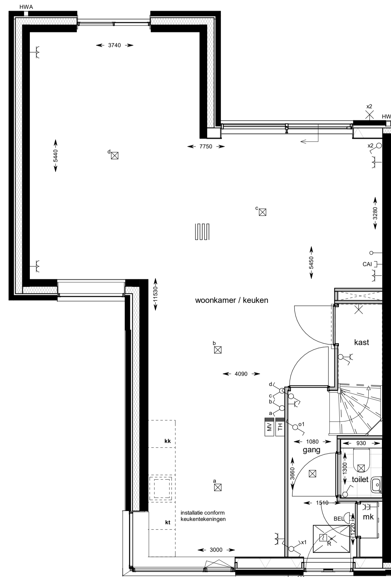
begane grond 1 : 50
