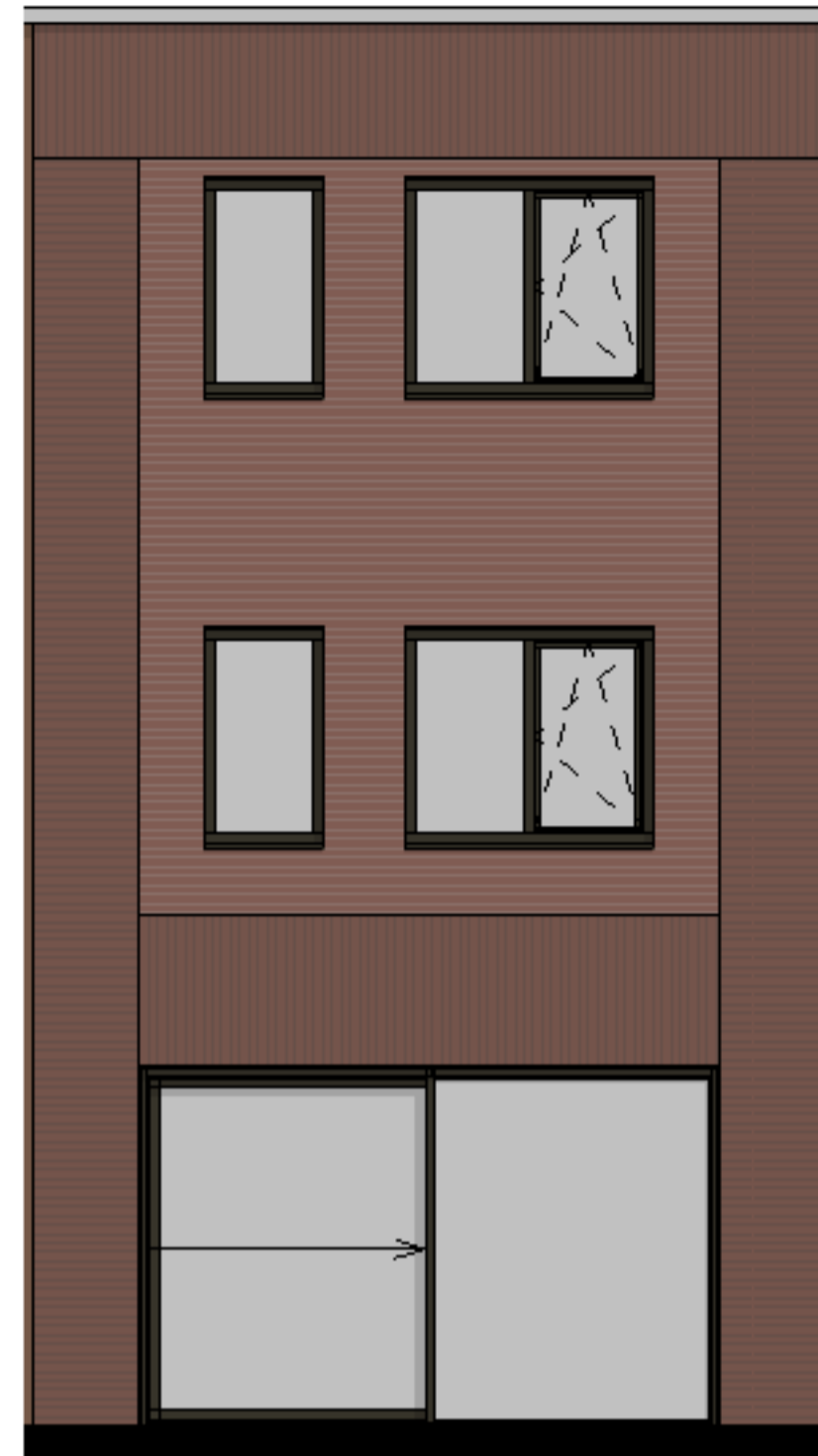
West binnengevel 1 : 50
