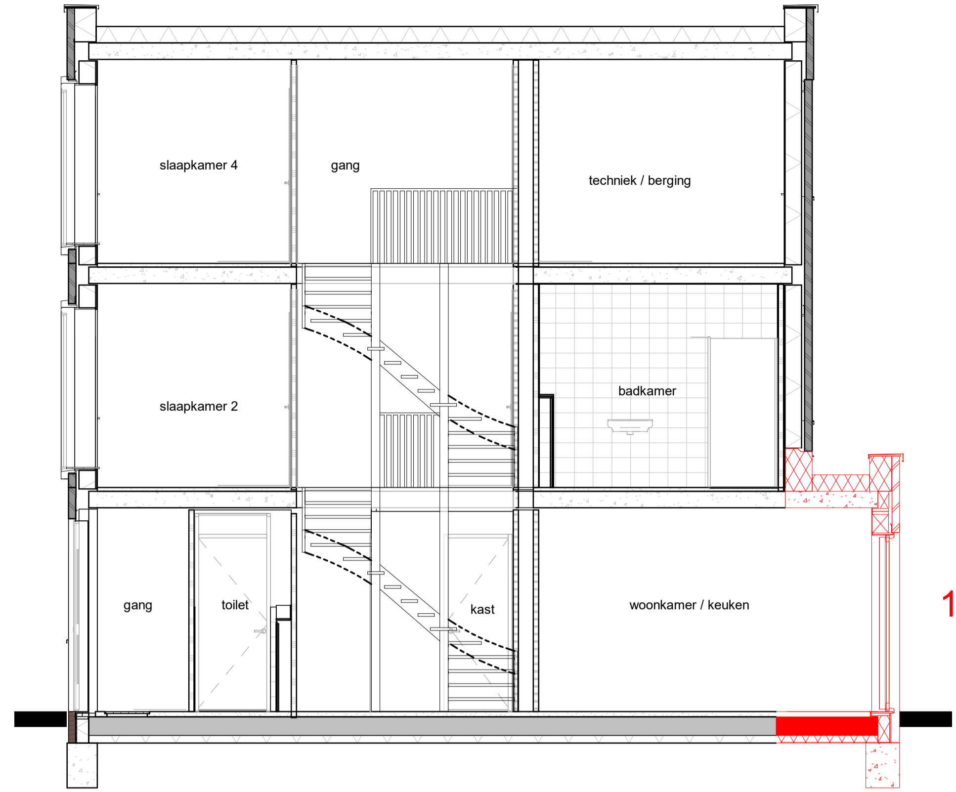
doorsnede A
