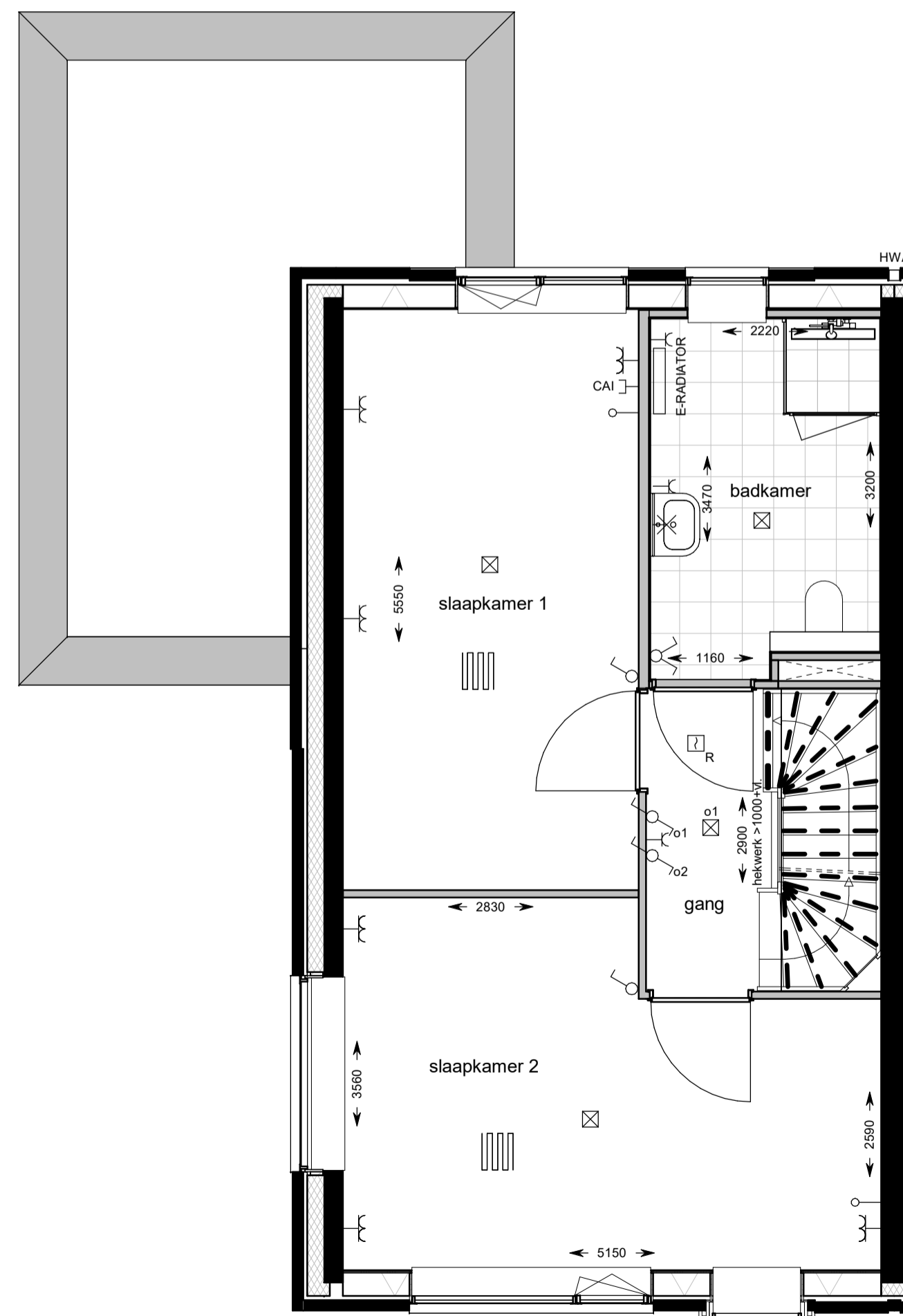
eerste verdieping 1 : 50
