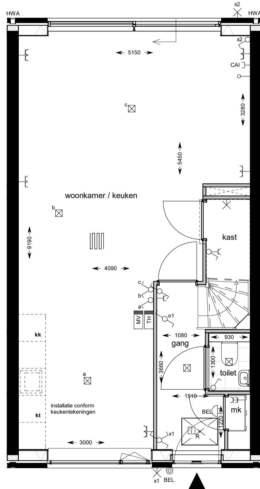
begane grond 1 : 50
