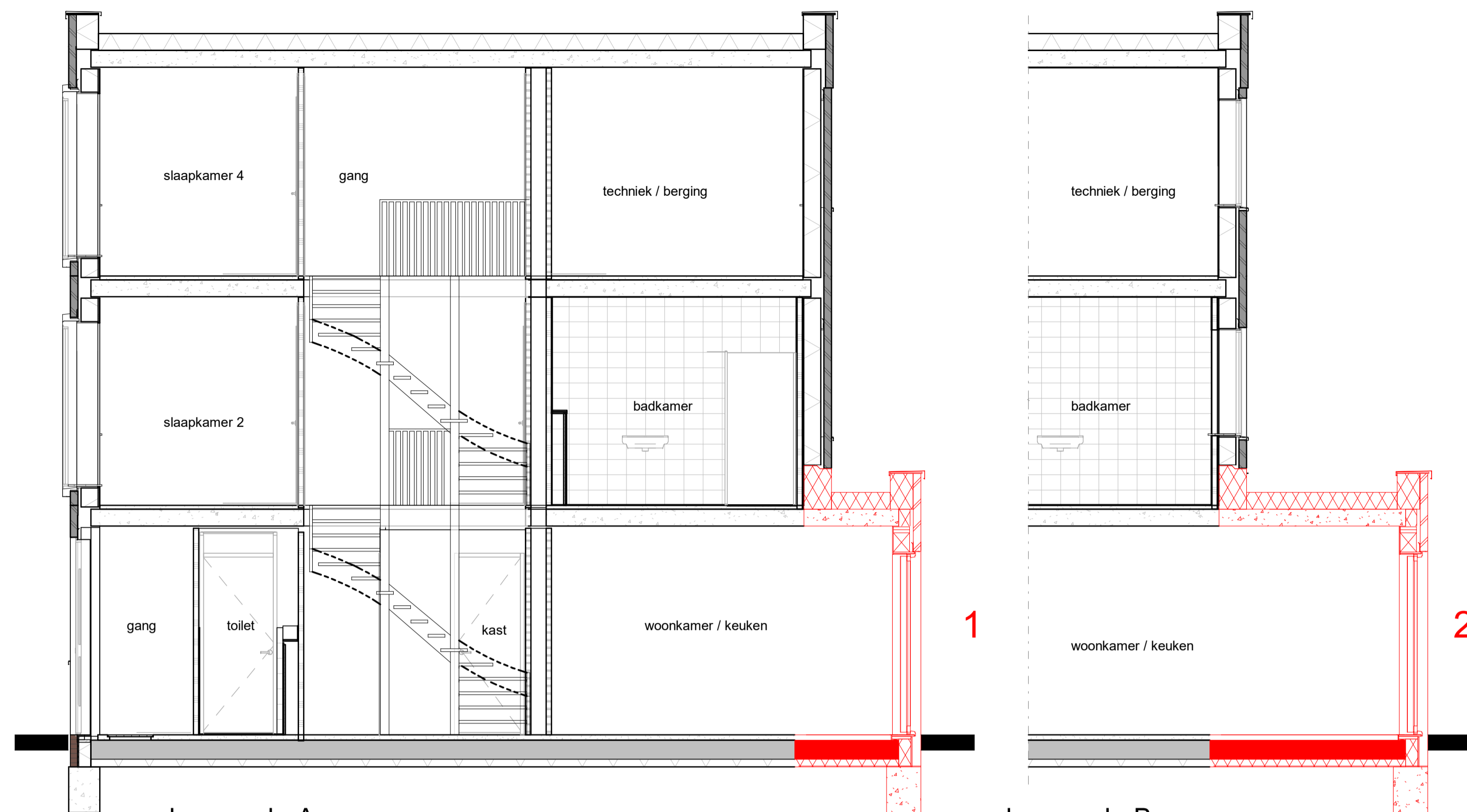
doorsnede A
