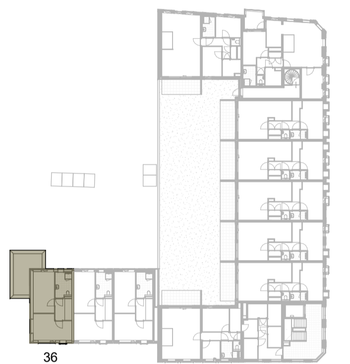
eerste/tweede verdieping
