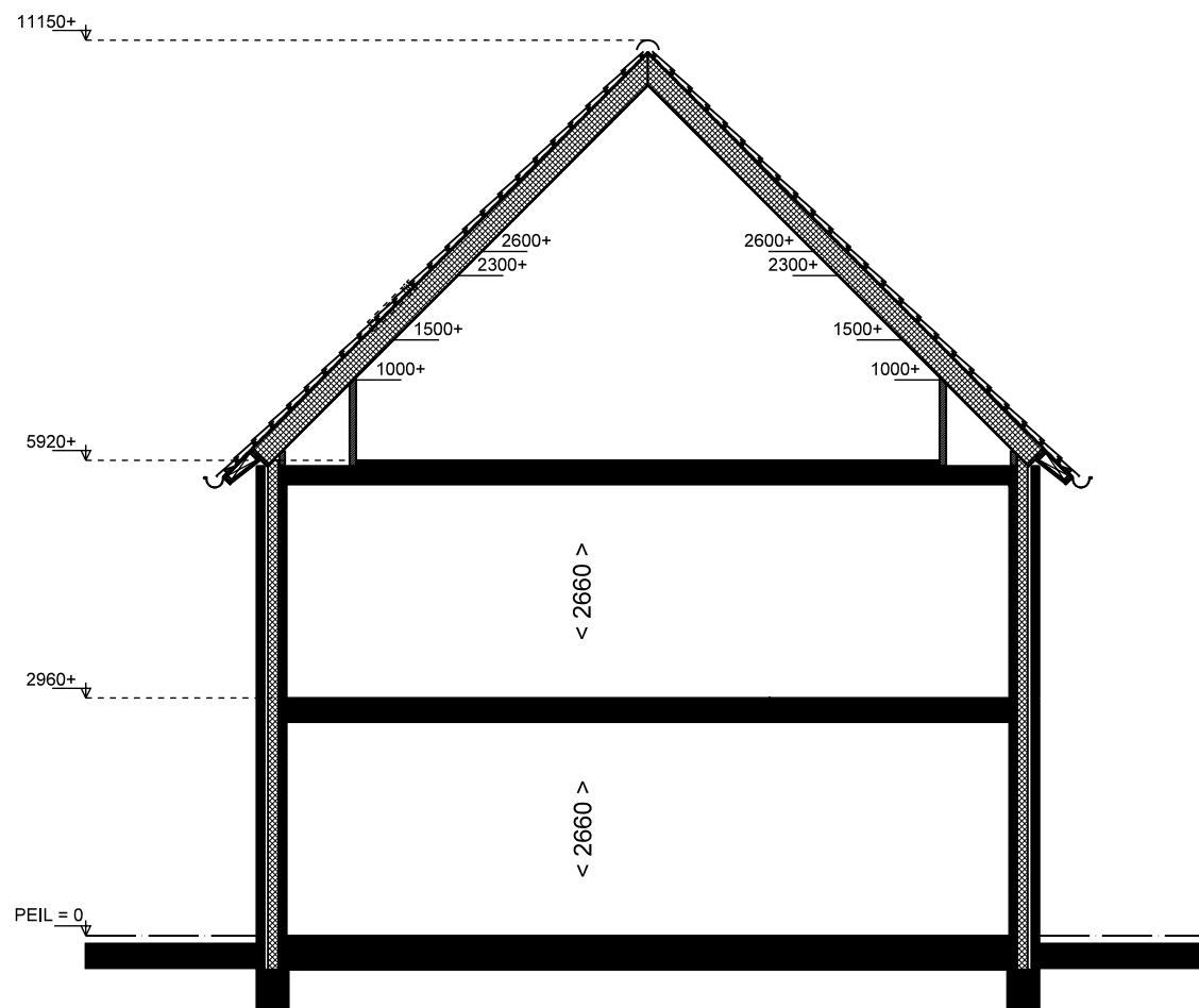
DOORSNEDE
