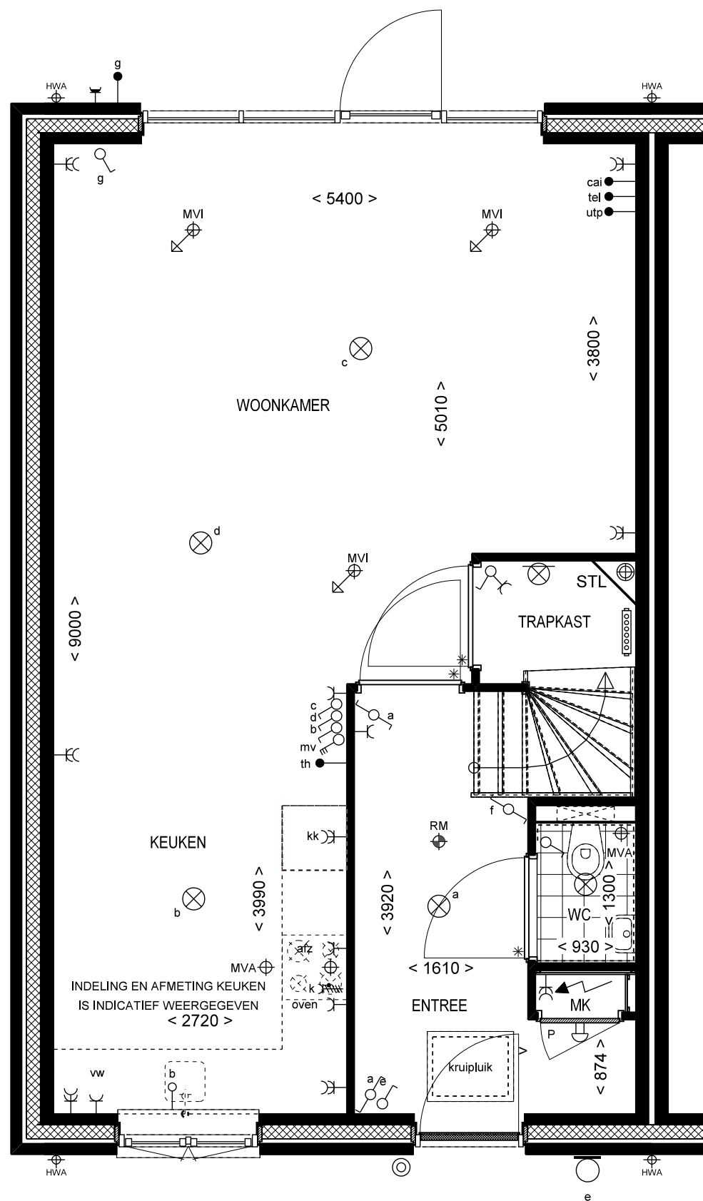
BEGANE GROND
