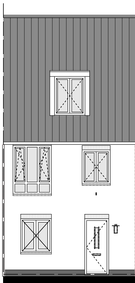
VOORGEVEL
