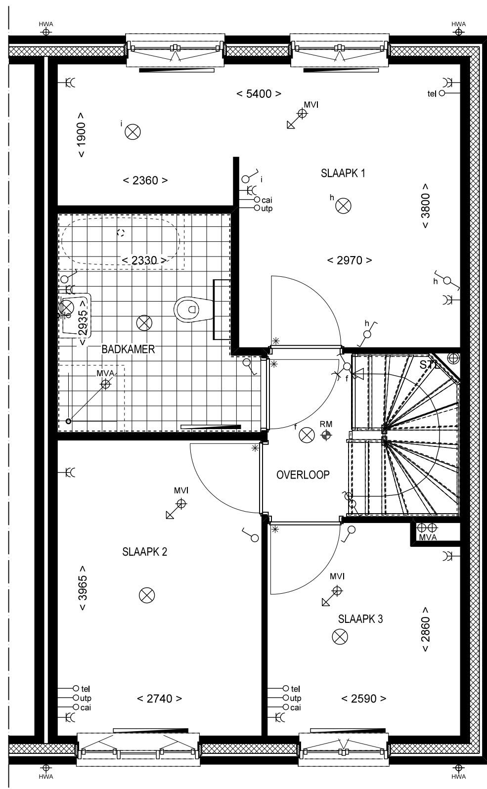
1e VERDIEPING
