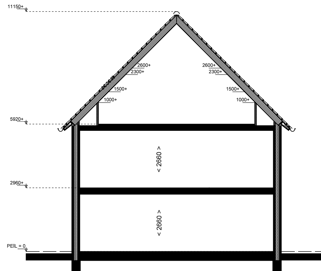
DOORSNEDE
