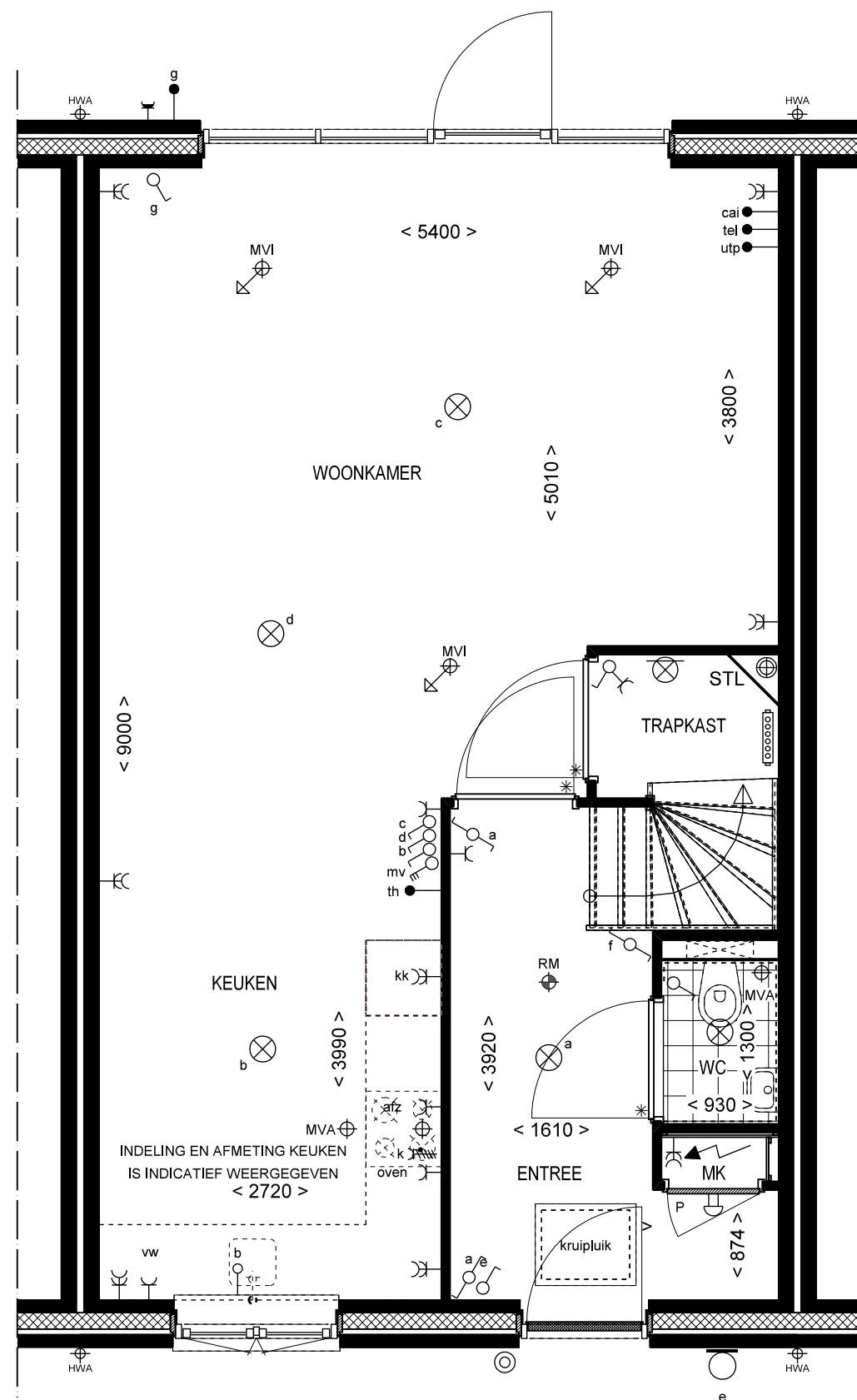
BEGANE GROND
