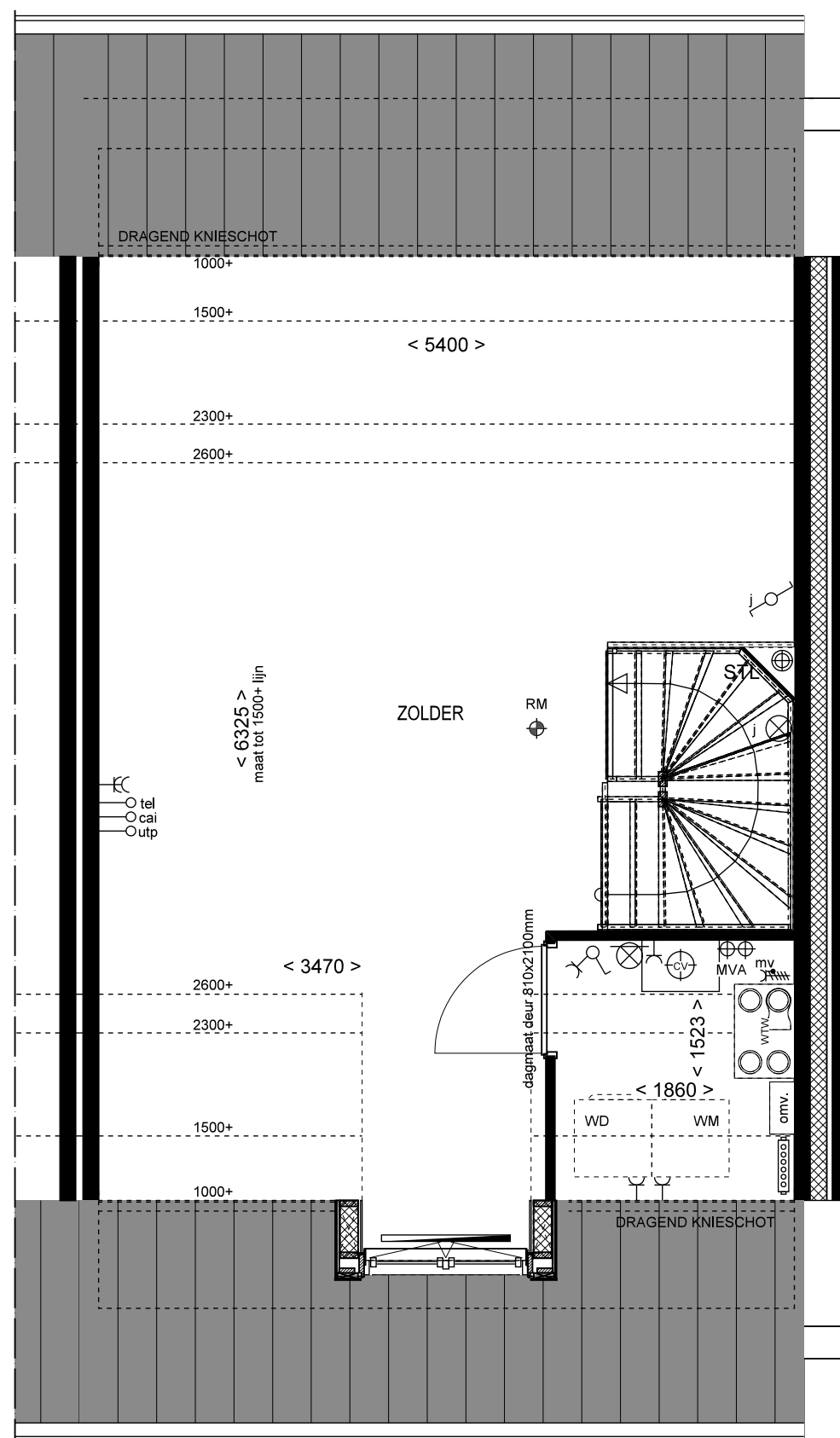
2e VERDIEPING
