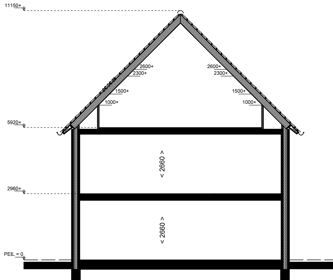
DOORSNEDE
