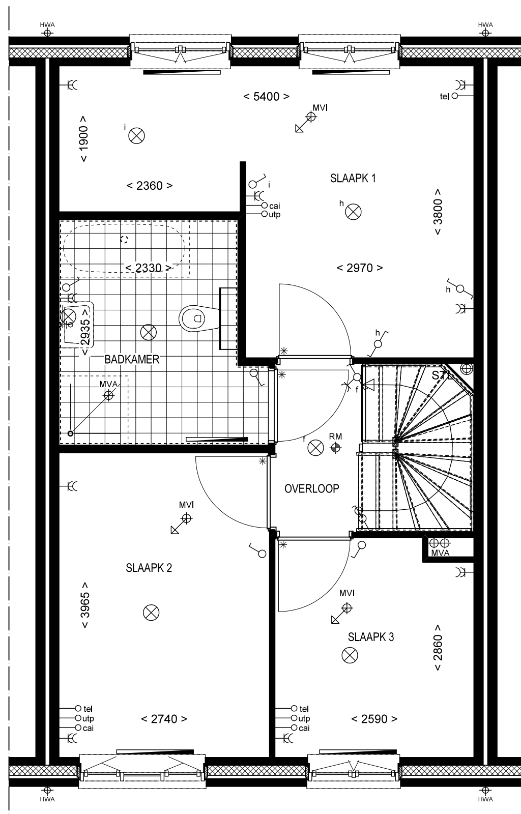
1e VERDIEPING
