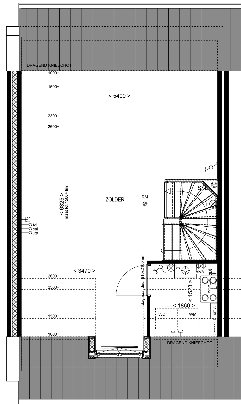
2e VERDIEPING
