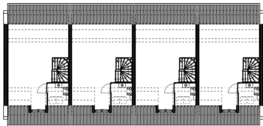
BNR 48 TYPE B1I BNR 47 TYPE B1 BNR 46 TYPE B1 BNR 45 TYPE B1r
