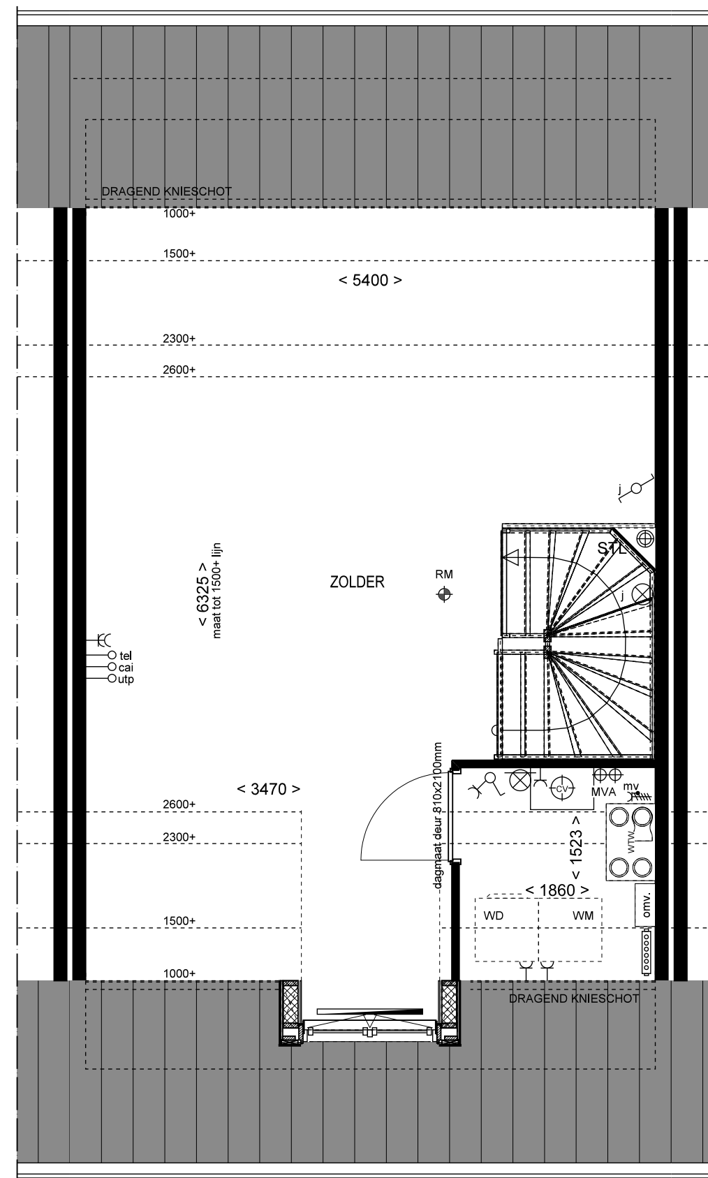
2e VERDIEPING
