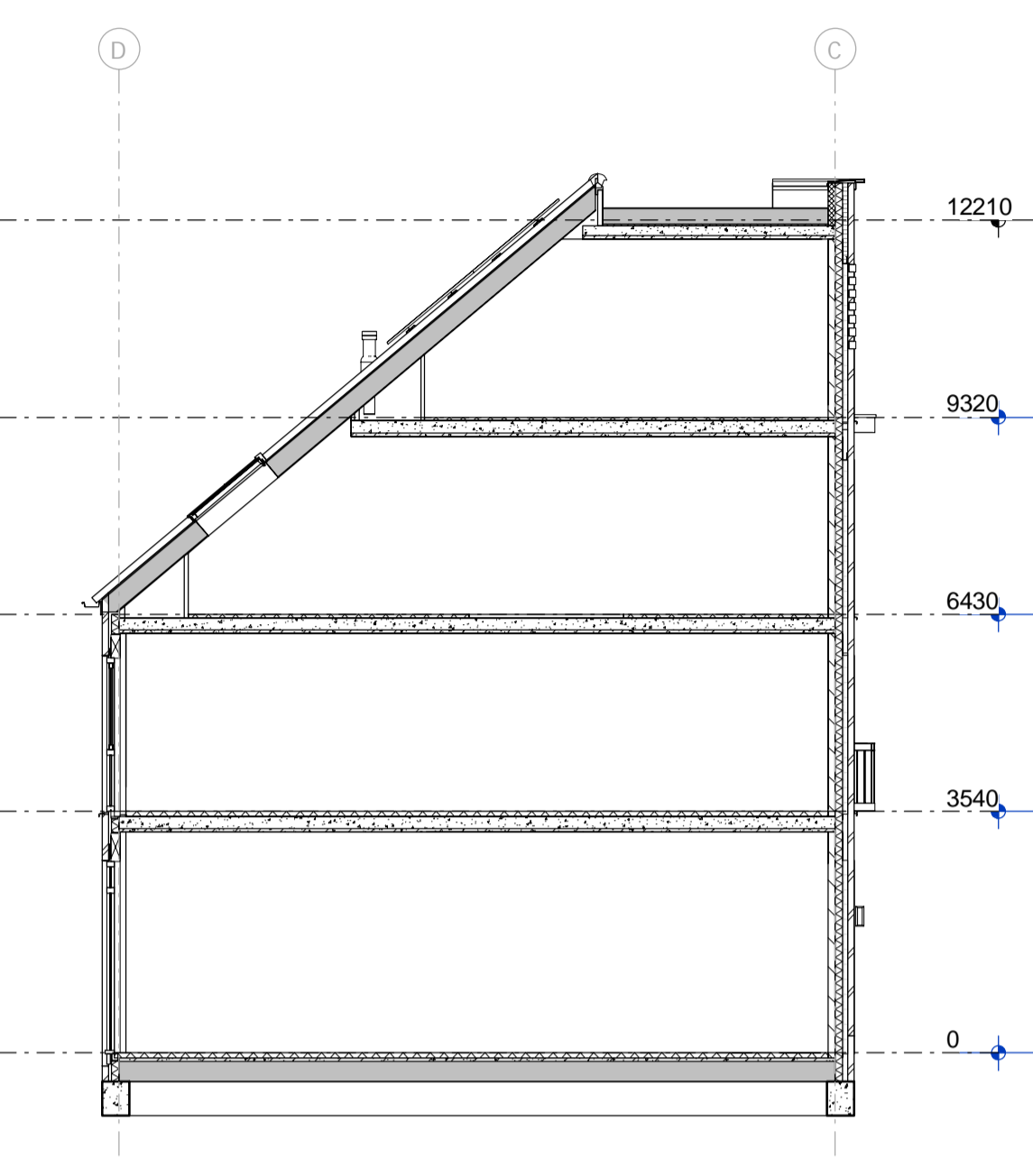
Doorsnede principe
