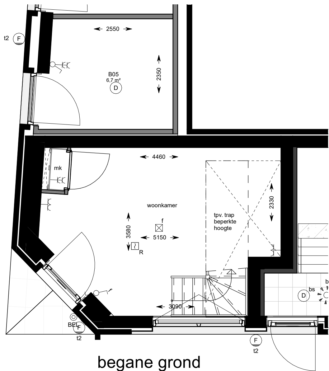
begane grond
