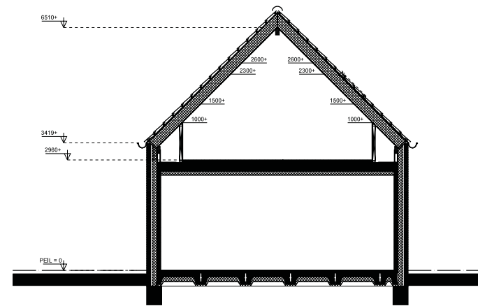
DOORSNEDE
