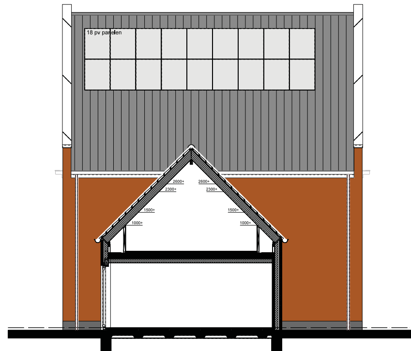
ZIJGEVEL
